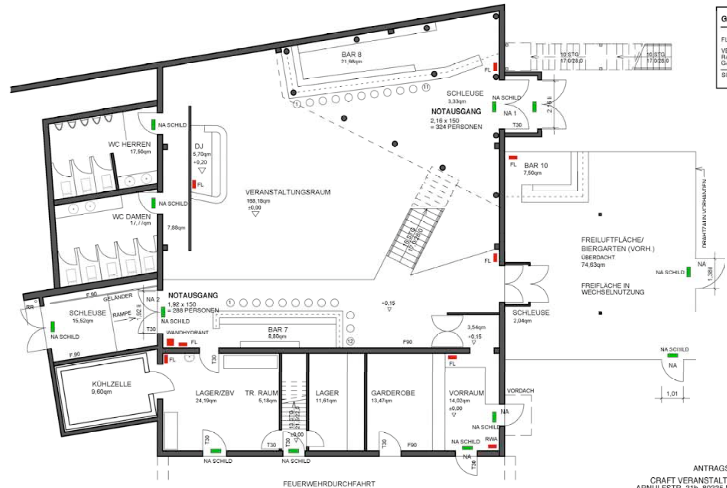
ERDGESCHOSS
