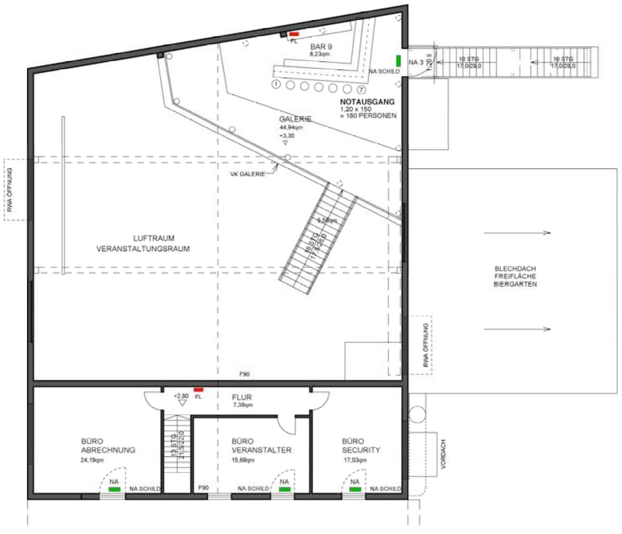
OBERGESCHOSS
